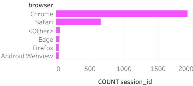
Browser Share
